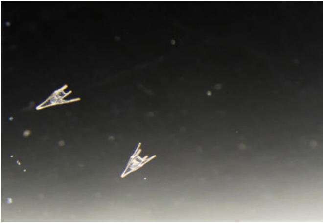
Fig- 4 - Saggi ecotossicologici, embriotossicità su Paracentrotus lividus (pluteo, 72h). L'immagine rappresenta due larve normoformate di echinoderma allo stadio di sviluppo di pluteo. La struttura caratteristica della larva a 72 ore dalla fecondazione risulta alterata morfologicamente nel caso in cui il campione di elutriato di sedimento nel quale vengono poste in incubazione le uova fecondate, sia tossico per questa specie
